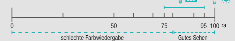
Grafik 1: Die Farbe des Lichts (Ra)
